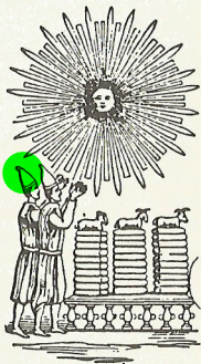
Ägyptisches Sonnenbild
