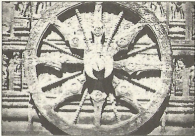
Babylonisches Sonnenrad
